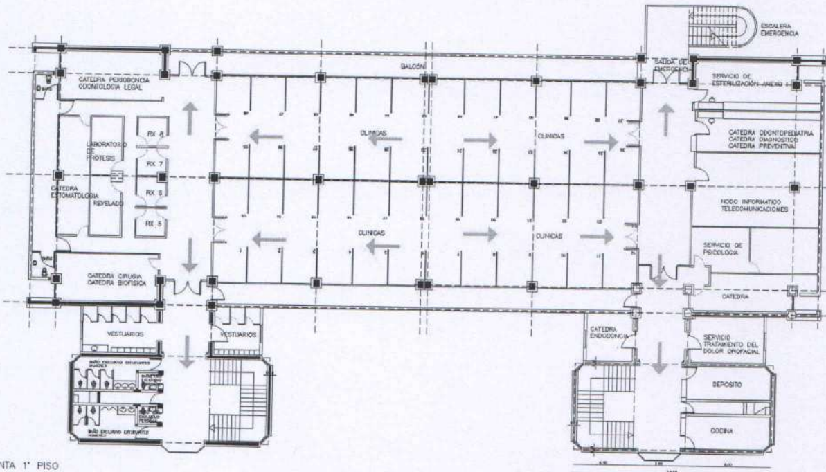
PLANTA 1º PISO
